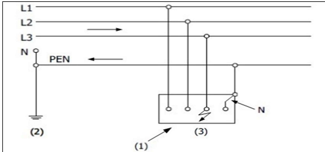
Figures 4.4. Boucle de défaut dans un schéma TN-C en courant alternatif et en courant continu
