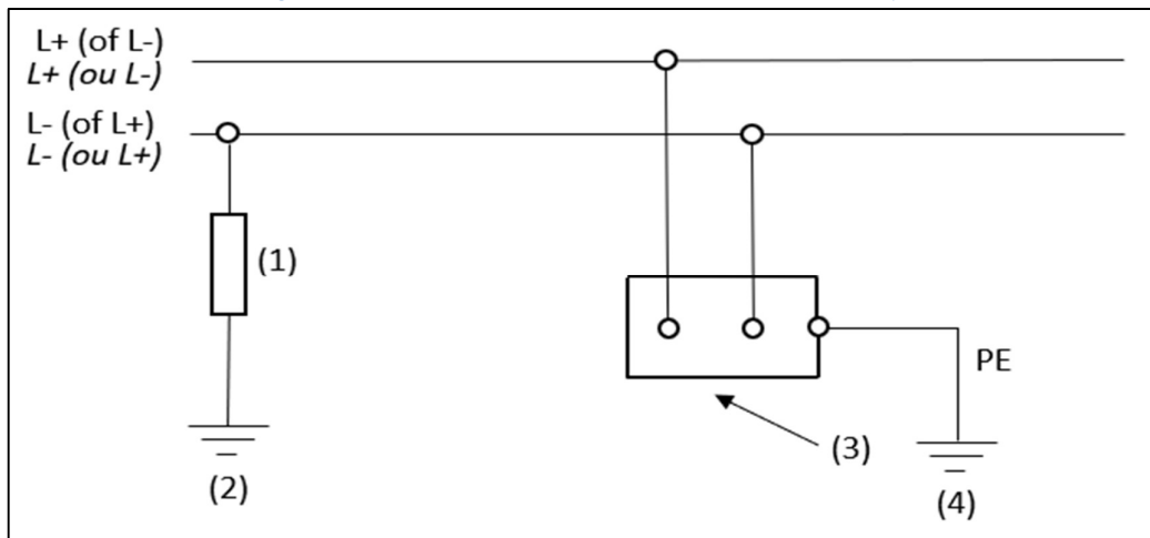
Figures 2.15. Schéma IT avec deux et trois conducteurs actifs
