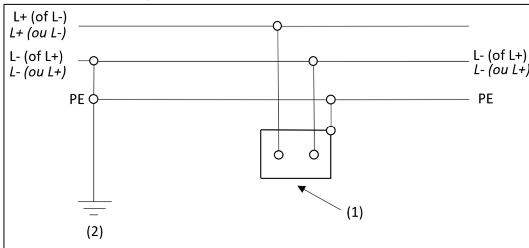
Figure 2.8. Schéma TN-S avec deux conducteurs actifs
