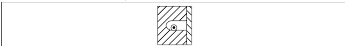
Figure 2.28. Mode de pose «moulure»
