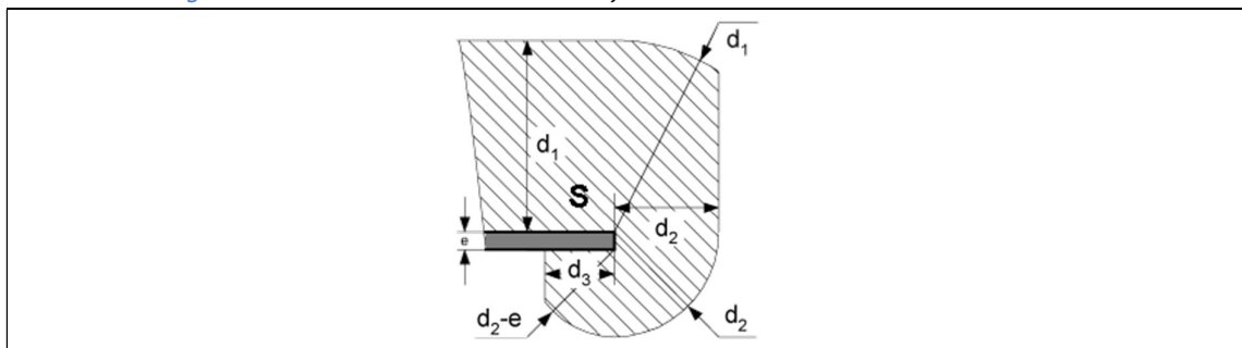
Figure 2.17. Volume d'accessibilité: la surface de circulation est limitée par un élément matériel
