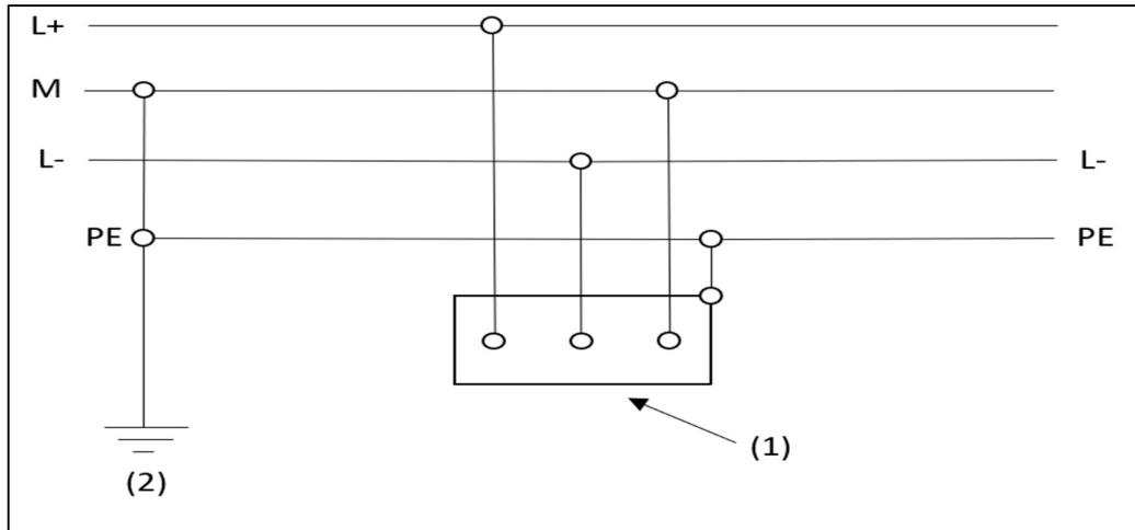
Figure 2.9. Schéma TN-S avec trois conducteurs actifs
