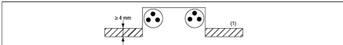
Figure 5.28. Coupe schématique d'une saignée
