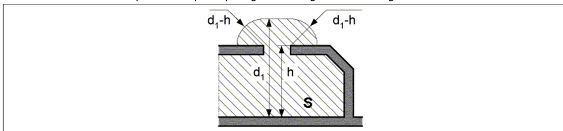
Figure 2.19. Volume d'accessibilité: des ouvertures existent dans les éléments matériels limitant la surface de circulation et ne permettent pas le passage d'une longue barre rectiligne de 12 mm de diamètre
