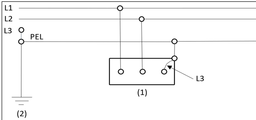
(1) Masse (2) Prise de terre du réseau
