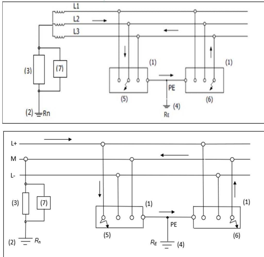
Figures 4.8. Schéma IT (deux défauts à la masse ou à la terre simultanés avec masses interconnectées) en courant alternatif et en courant continu
