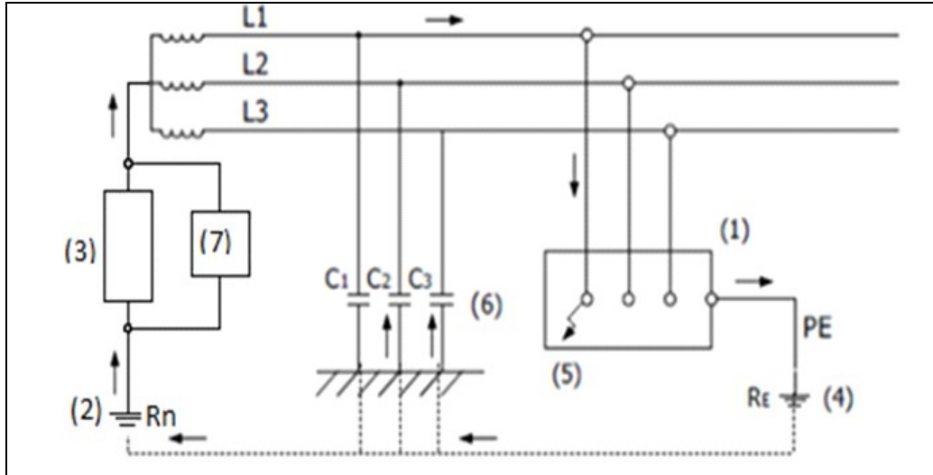
Figures 4.7. Schéma IT (premier défaut à la masse ou à la terre) en courant alternatif et en courant continu
