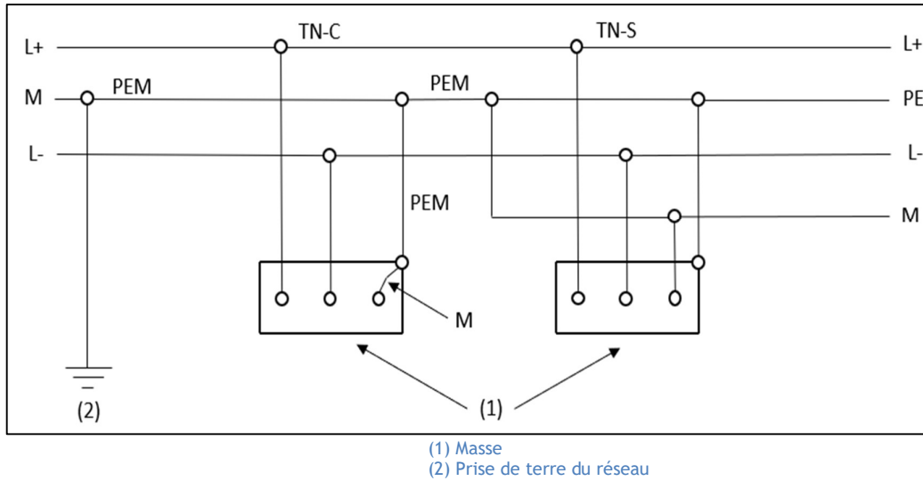
Figure 2.13. Schéma TN-C-S avec trois conducteurs actifs
