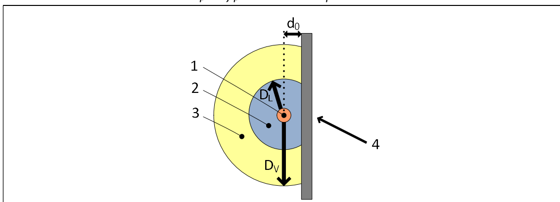
Figure 2.33. Représentation de la zone sous tension et de la zone de voisinage avec dispositif protecteur métallique mis à la terre
