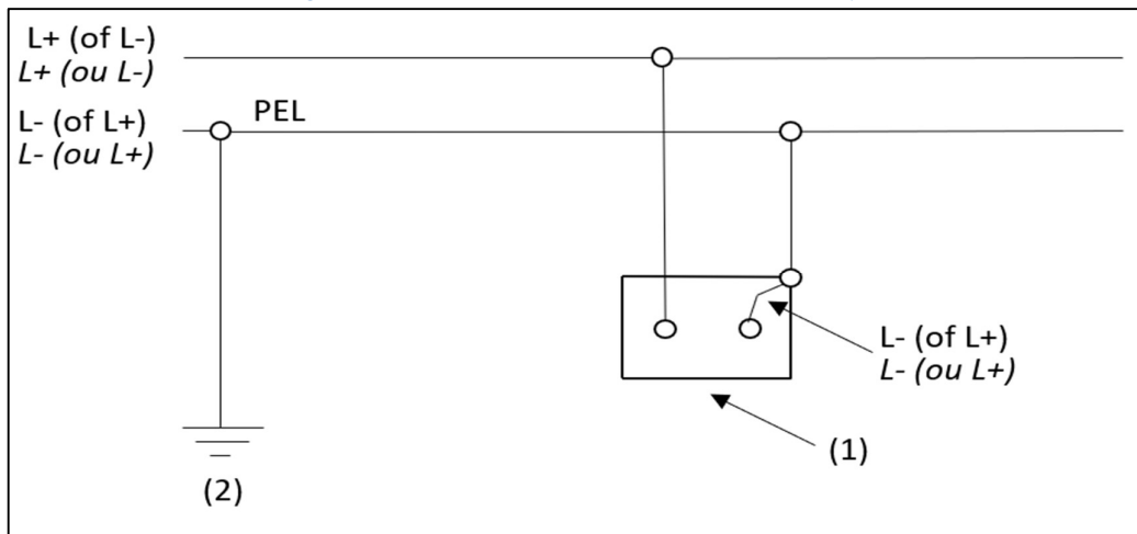
Figure 2.10. Schéma TN-C avec deux conducteurs actifs
