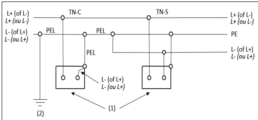
Figure 2.12. Schéma TN-C-S avec deux conducteurs actifs
