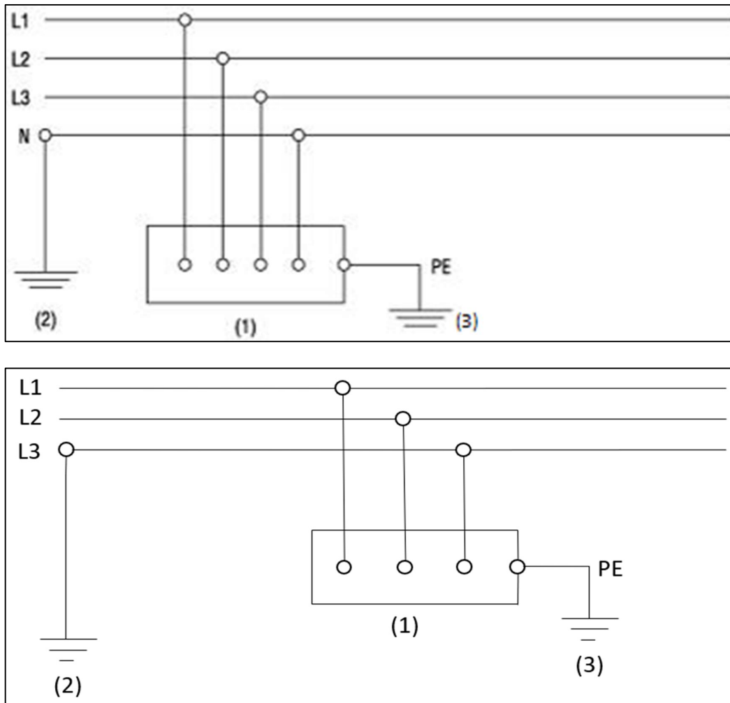
Figure 2.4. Schéma TT
