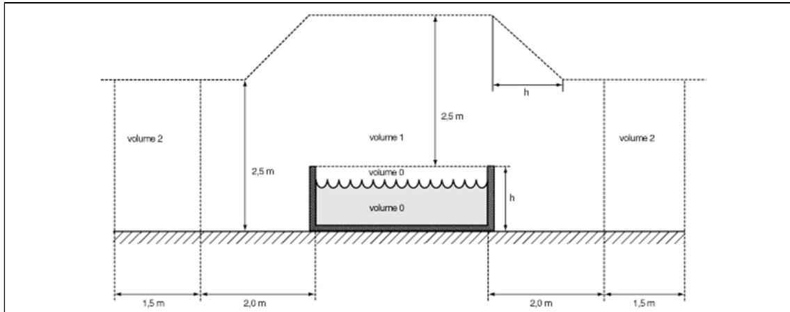
Figure 7.14. Piscines: exemple de dimensions de volumes avec cloisons fixes d'au moins 2,5 m de hauteur (représentation plane)
