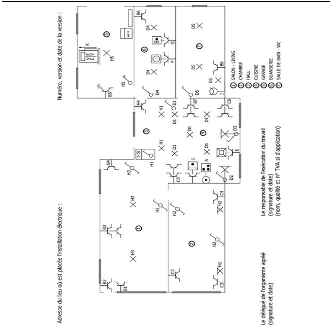
Figure 3.2. Exemple de plan de position
