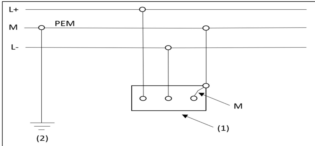
Figure 2.11. Schéma TN-C avec trois conducteurs actifs
