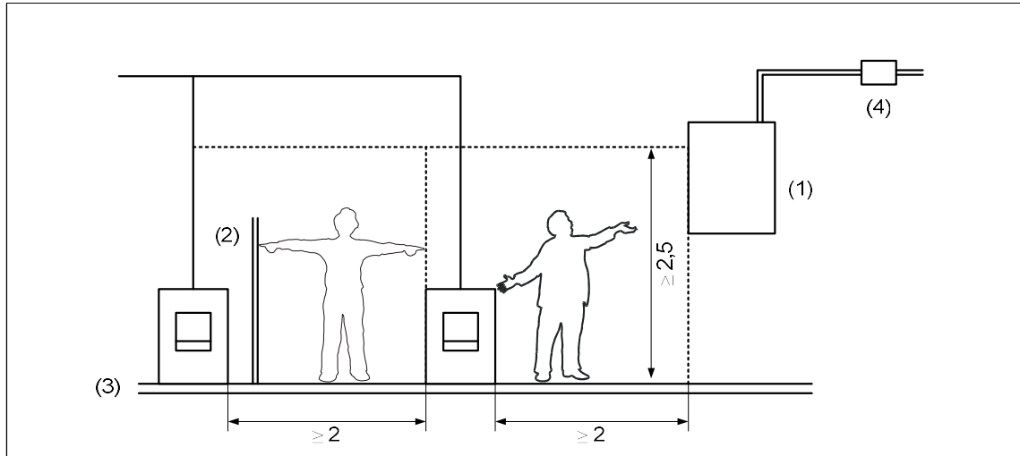
Figure 4.2. Protection rendant impossible le contact simultané entre pièces susceptibles d'être portées à des potentiels dont la différence est dangereuse (2)
