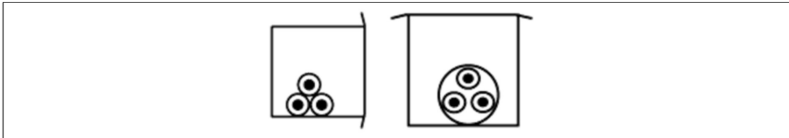
Figure 2.25. Mode de pose «goulotte»
