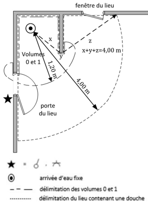
g.2. Local contenant une douche, avec des parois verticales fixes toutes d'une hauteur d'au moins 2,25 m ou avec des parois verticales fixes qui sont toutes jointives avec un plafond ou, si présent, un faux plafond qui n'est pas ajouré ou démontable sans l'aide d'un outil
