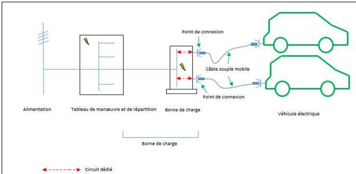
Figure 7.20. Borne de charge avec deux points de connexion « socles de prise de courant sur borne de charge » faisant partie de la borne de charge (dispositifs de protection contre les surintensités des circuits dédiés intégrés dans la borne de charge)
