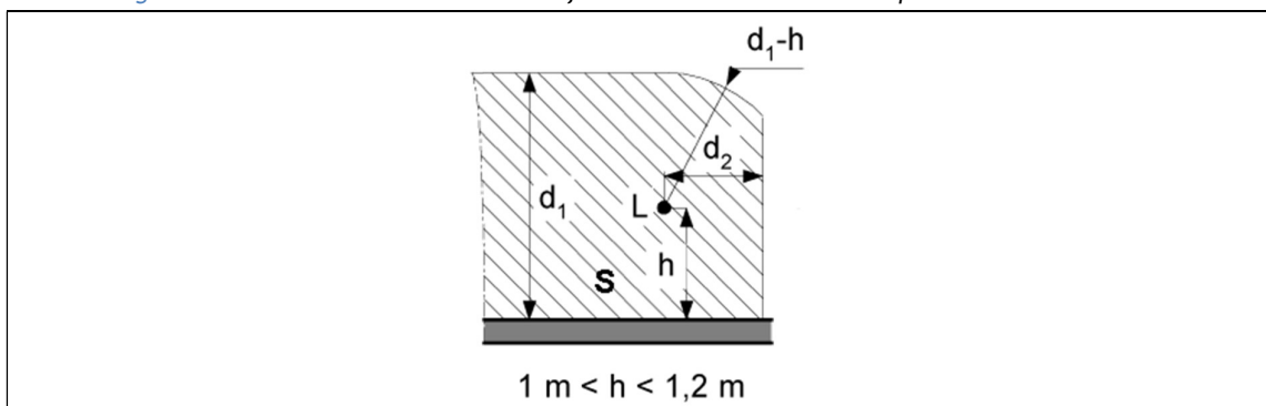
Figure 2.17. Volume d'accessibilité: la surface de circulation est limitée par un élément matériel
