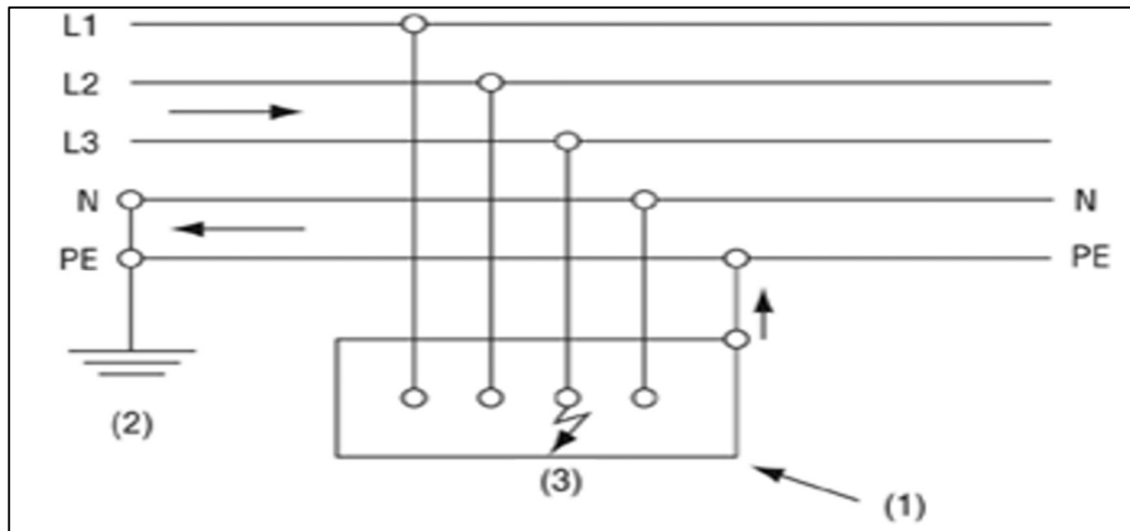
Figures 4.3. Boucle de défaut dans un schéma TN-S en courant alternatif et en courant continu
