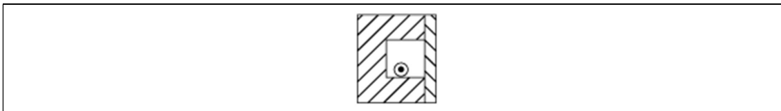
Figure 2.29. Mode de pose «plinthe rainurée (ou chambranle)»
