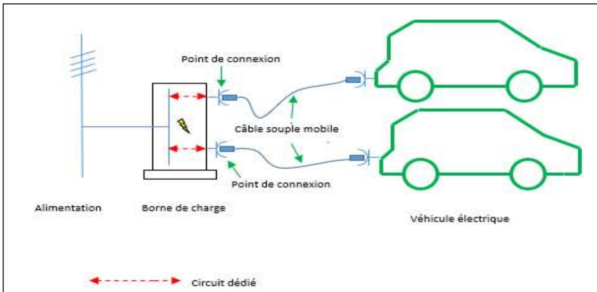
Figure 7.18. Borne de charge avec deux points de connexion « socles de prise de courant sur borne de charge » faisant partie de la borne de charge (dispositifs de protection contre les surintensités des circuits dédiés intégrés dans la borne de charge)
