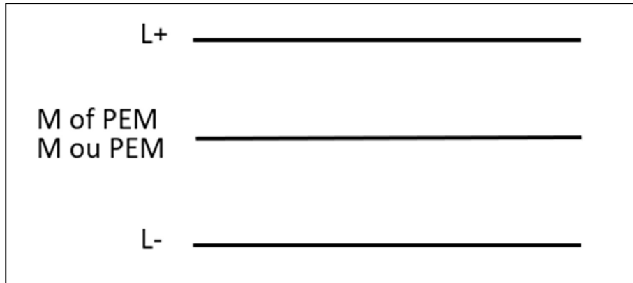
Figure 2.7. Schéma mis à la terre en courant continu avec trois conducteurs actifs
