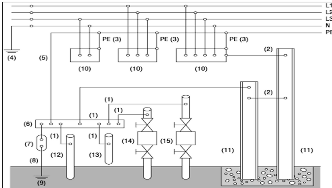
Figures 2.20. Installation de mise à la terre en courant alternatif et en courant continu
