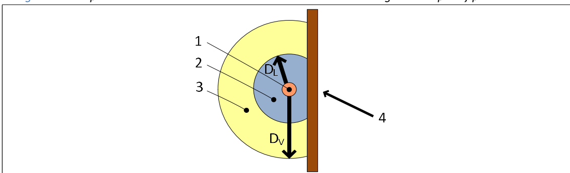
Figure 2.32. Représentation de la zone sous tension et de la zone de voisinage avec dispositif protecteur isolant
