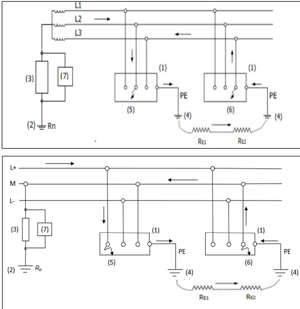
Figures 4.9. Schéma IT (deux défauts à la masse ou à la terre simultanés avec masses non interconnectées) en courant alternatif et en courant continu
