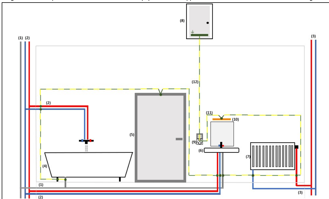
Figure 7.1. Exemple d'installation de la liaison équipotentielle supplémentaire dans un lieu contenant une baignoire
