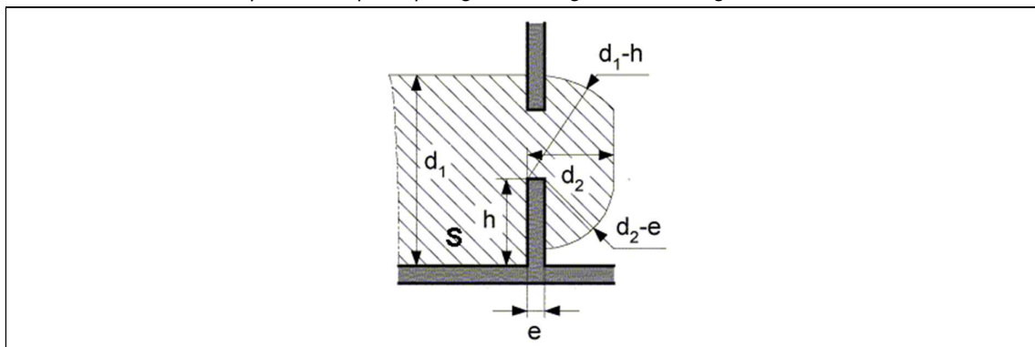
Figure 2.19. Volume d'accessibilité: des ouvertures existent dans les éléments matériels limitant la surface de circulation et ne permettent pas le passage d'une longue barre rectiligne de 12 mm de diamètre
