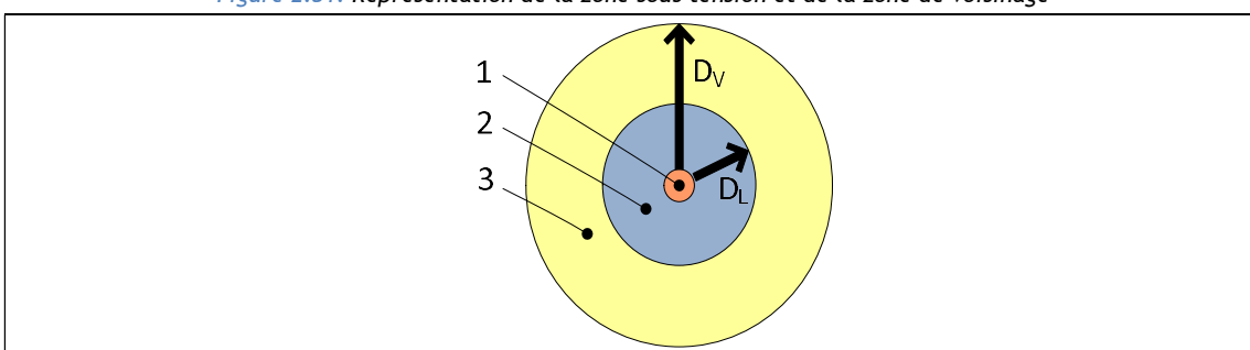
Figure 2.31. Représentation de la zone sous tension et de la zone de voisinage
