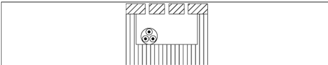
Figure 2.22. Mode de pose «caniveau ou gaine de sol»
