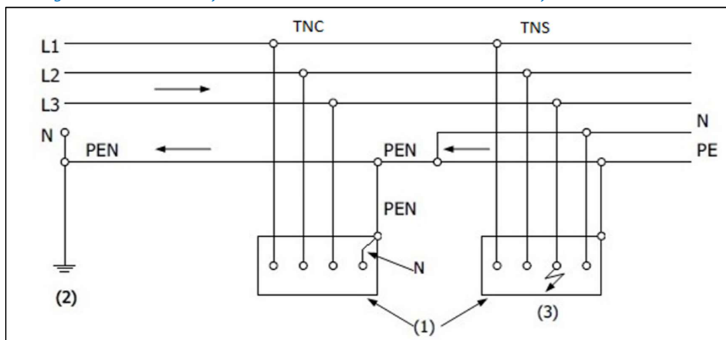
Figures 4.5. Boucle de défaut dans un schéma TN-C-S en courant alternatif et en courant continu
