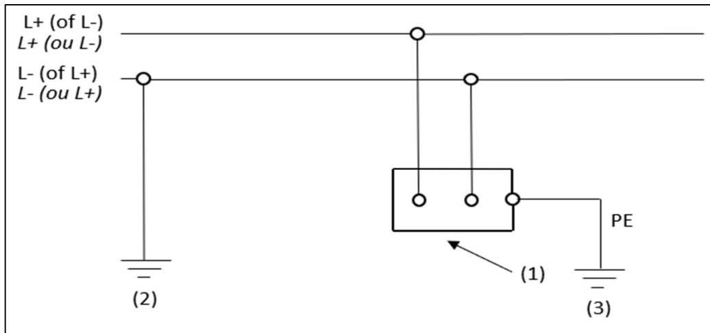
Figures 2.14. Schéma TT avec deux et trois conducteurs actifs
