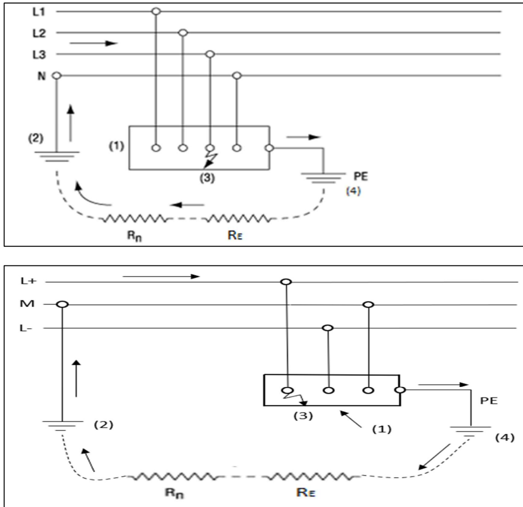
Figures 4.6. Boucle de défaut dans un schéma TT en courant alternatif et en courant continu
